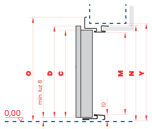
PRZEKRÓJ PIONOWY
