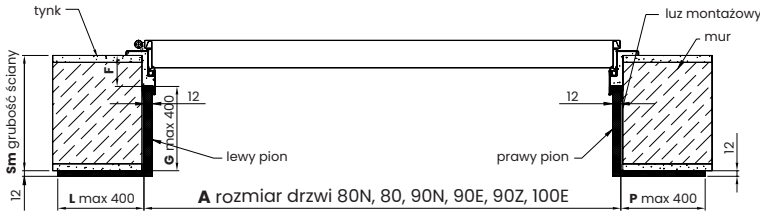
PRZEKRÓJ POZIOMY
