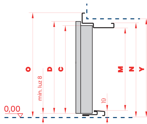
PRZEKRÓJ PIONOWY
